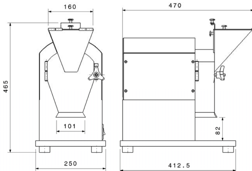
Martillo triturador con criba intercambiable.
